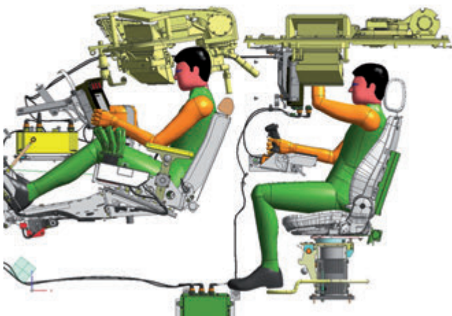
werkplek van bestuurder en mineur
