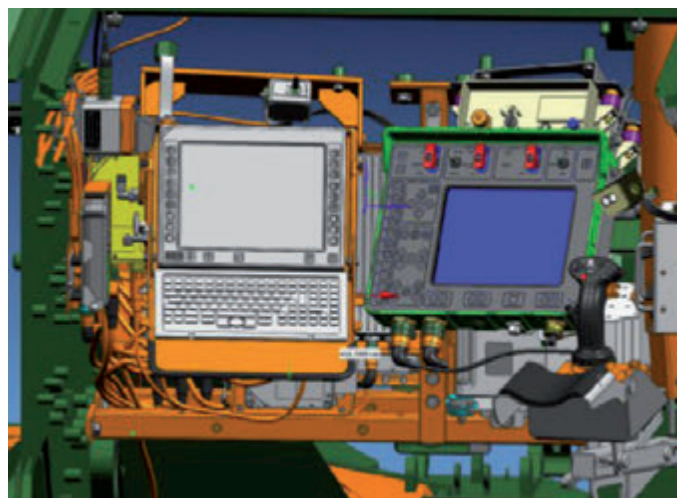
werkplek van de commandant met BMS, DCP en ITS
